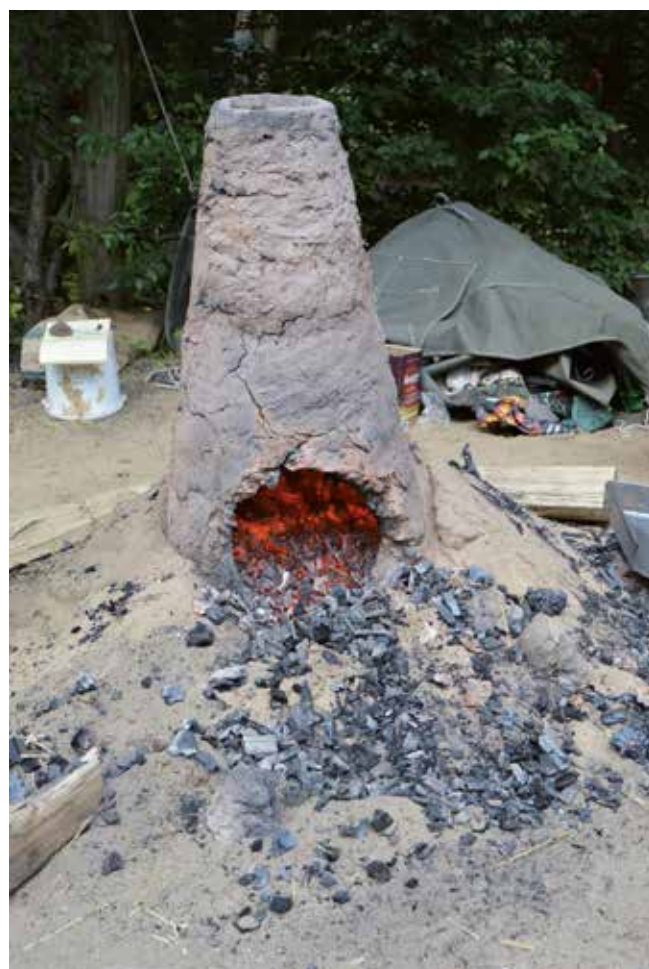
Obr. 4: Šachtová kusová železářská pec po tavbě. Foto N. Belisová
