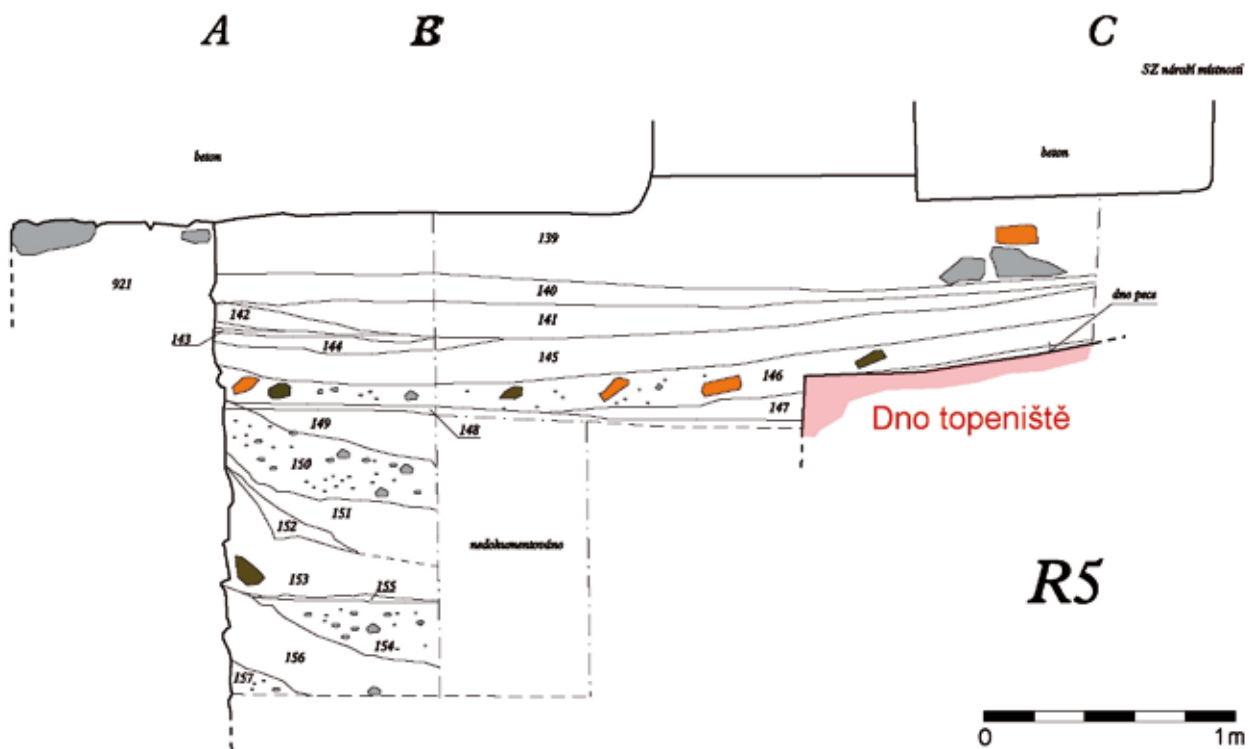
Obr. 3: Řez (R5) pyrotechnickým zařízením v rámci někdejší kuchyně
