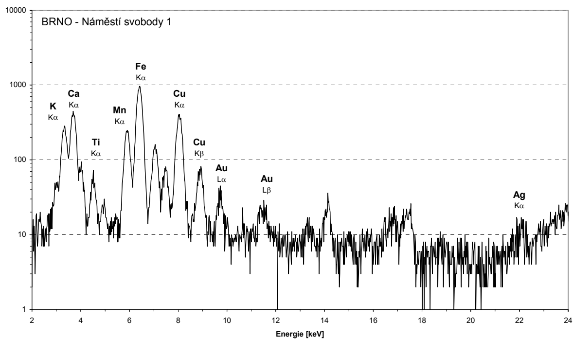
Obr. 7 XRF spektrum červeně zbarvené skloviny na povrchu tyglíku Brno NS 1
